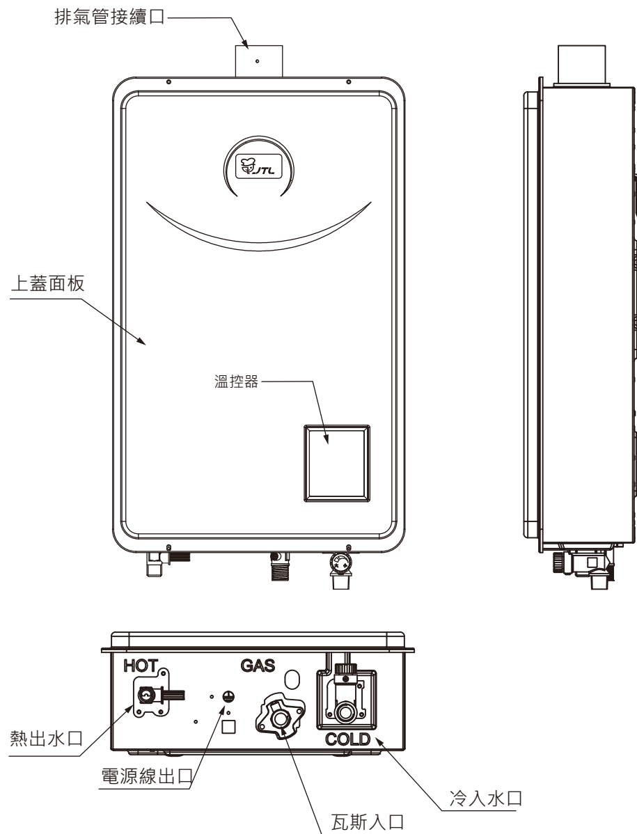
外觀：(JT-H1632/H1636/H1622/H1652/H1655/H1332/H1322)
