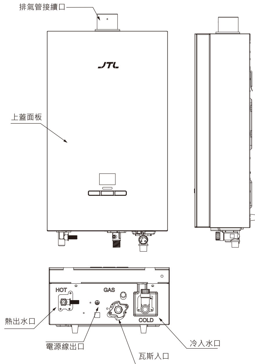
外觀：(JT-H1635/H1335)
